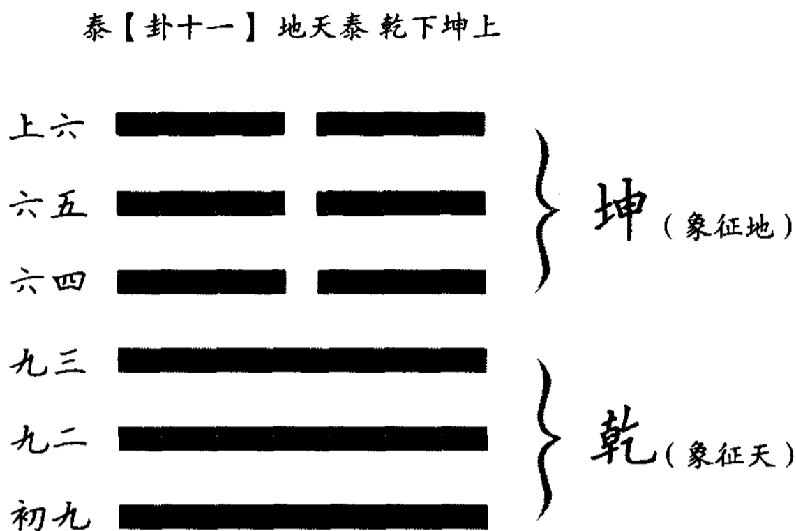
图1-泰卦示意图
