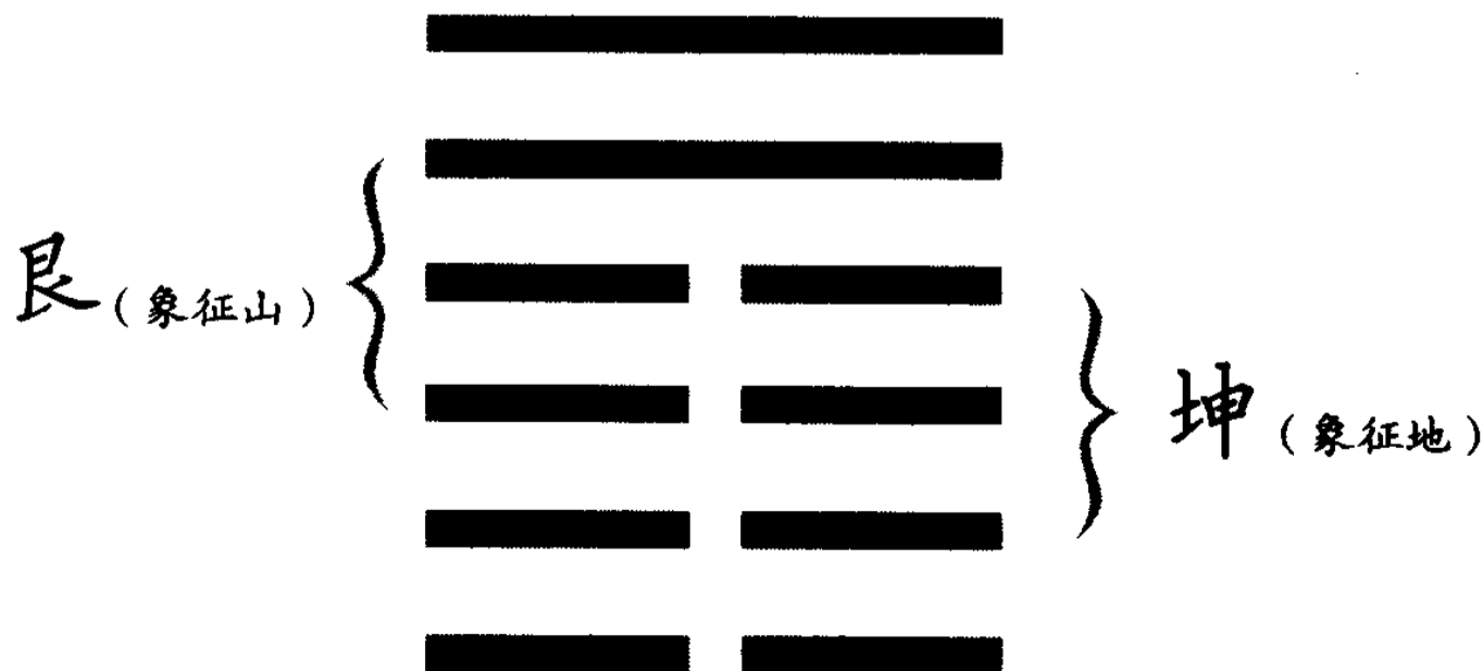
图 16 - 观卦的互体
